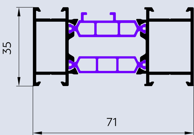
СТ 7138 Добор 35 мм
