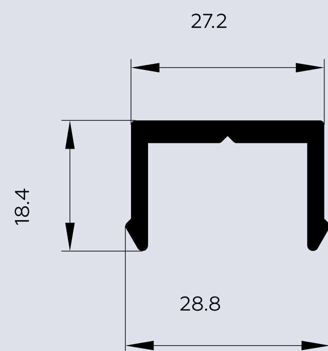
КПС 1521 Соединитель рам
