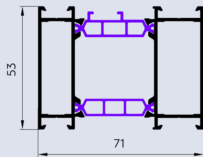
СТ 7139 Добор 53 мм
